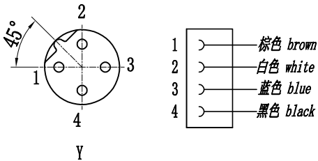
针位图 Contact arrangements 接线图 Circuit diagram
